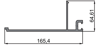
• 10-10097 • Polikarbon Taşıyıcı Profil/Polycarbonate Carrier Profile • 1.851 kg/m
