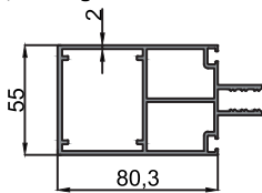
10-10100 Taşıyıcı Profil Yan Kapağı / Carrier Profile Side Cover 0.659 kg/m
