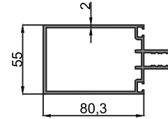
• 10-10097 • Polikarbon Taşıyıcı Profil/Polycarbonate Carrier Profile • 1.851 kg/m
