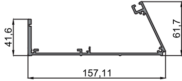
10-10284 Oluk Profili Dış Kapağı/Gutter Profile Outside Cover 1.402 kg/m
