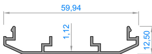
2580 - 0,324 kg/m
