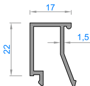
1152 - 0,298 kg/m
