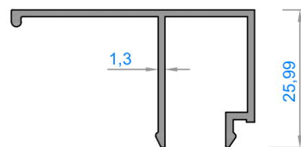
* 4503 - 0,361 kg/m
