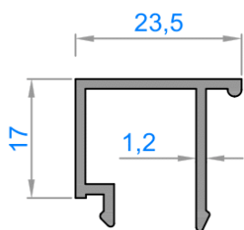
1151 - 0,232 kg/m
